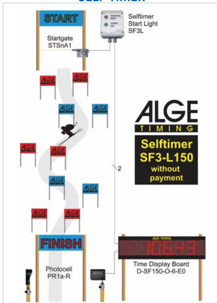
FEU DE DÉPART Contrôle du flux des participants REF SF3L
